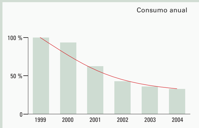
Consumo de energía en la destilación
